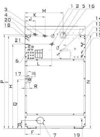
ARRIERE
